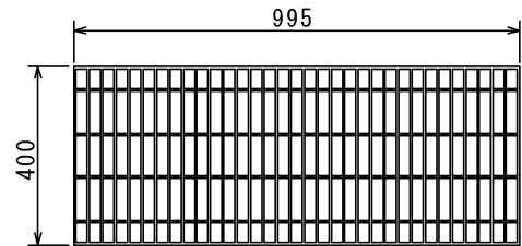
グレーチング詳細図 ※t=32mm
