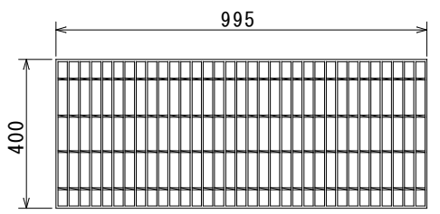
グレーチング詳細図
