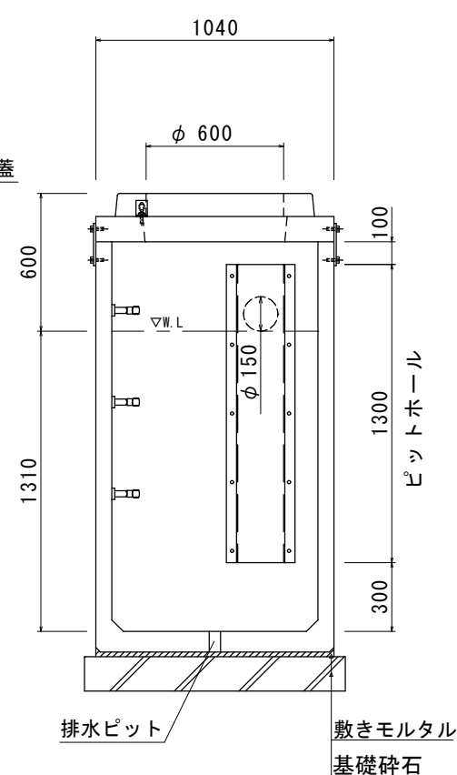
A-A断面図
