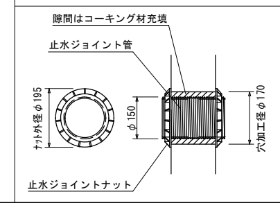
止水ジョイントパイプφ150
