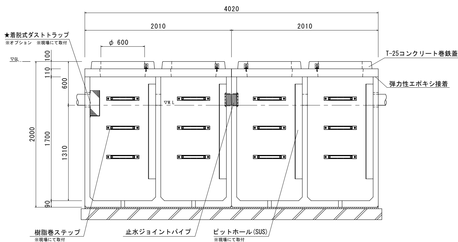
B-B断面図
