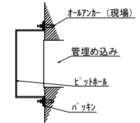
流出側ビットホル取付詳細図
