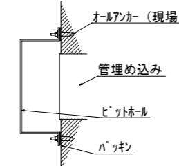
流出側ヒットホール取付詳細図
