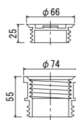
排水ヒット(栓付)詳細図
