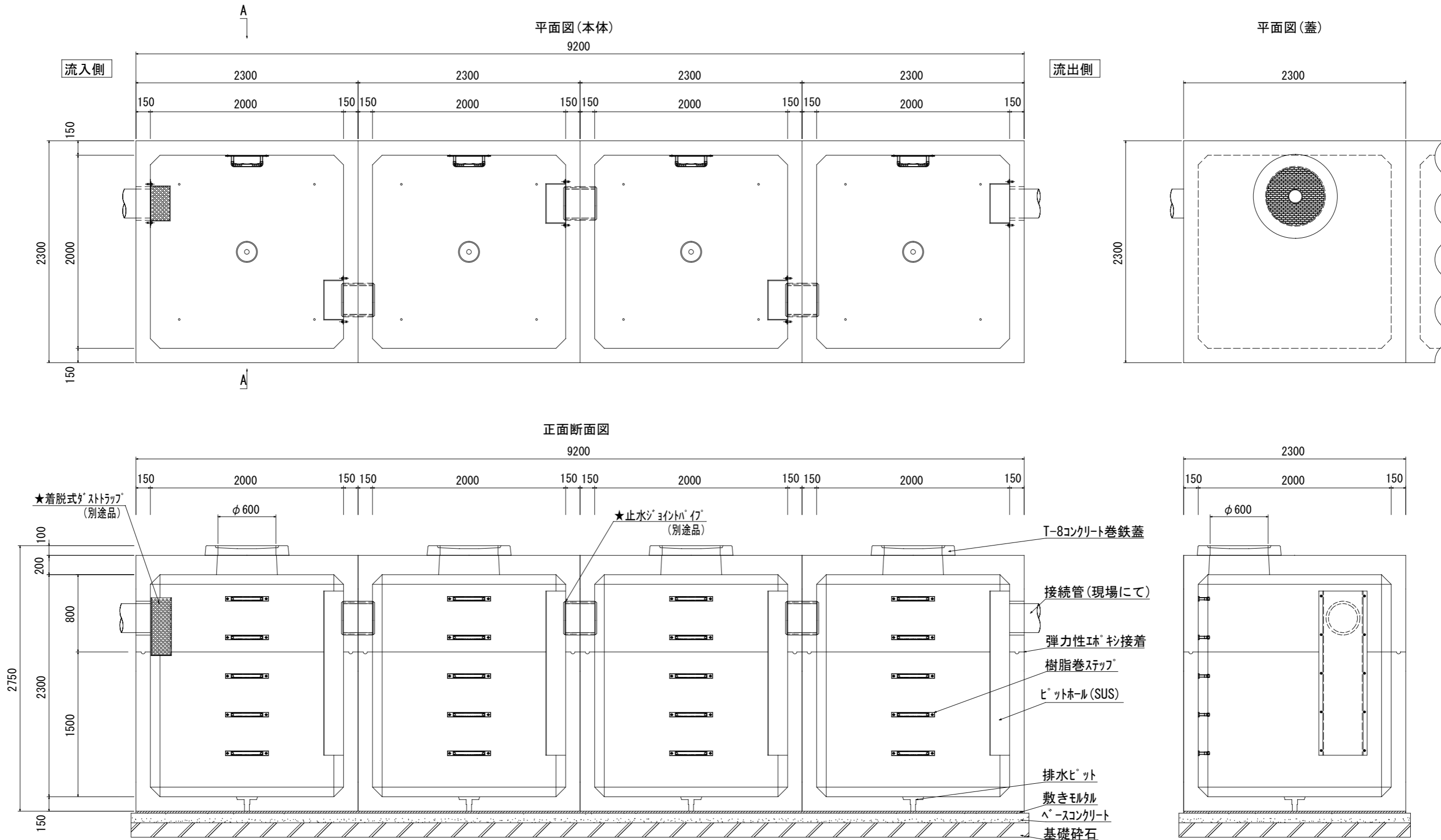
排水ヒット(栓付)詳細図
