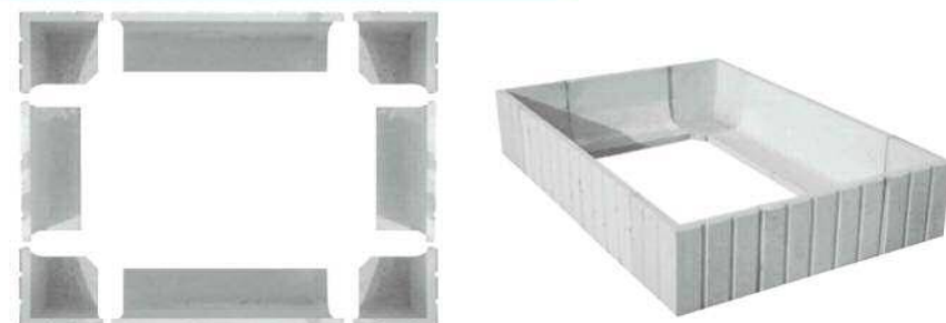
4 L1600×W1100 (①×2個+②×2個+③×4個)
