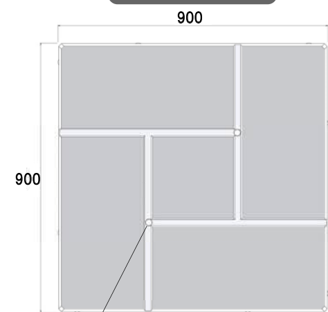
製品図面 (平面図)
