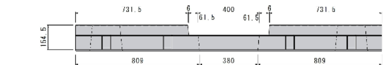
歩車道境界ブロック 両面 B
