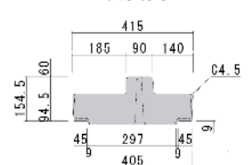
側面図
