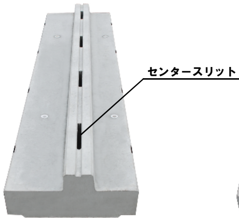
平面図（標準タイプ）
