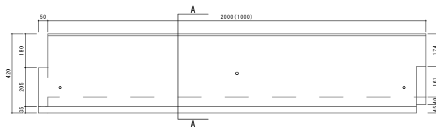
側面図
