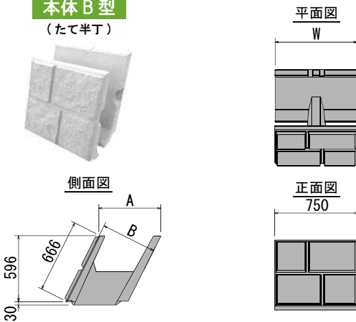
本体 B 型
