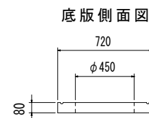
車道用鉄蓋 (H110)
