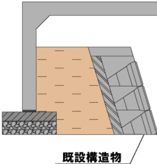
門型カルバート等
