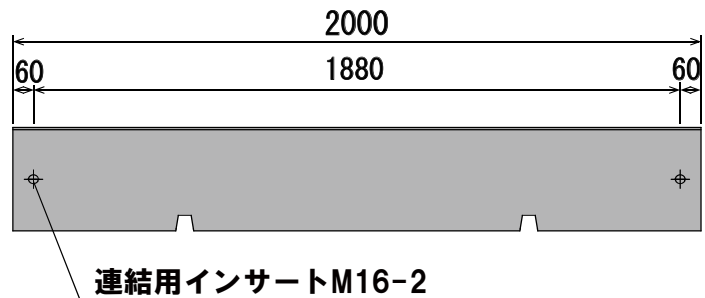
正面図
