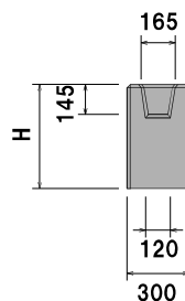
A矢視
