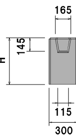
B矢視
