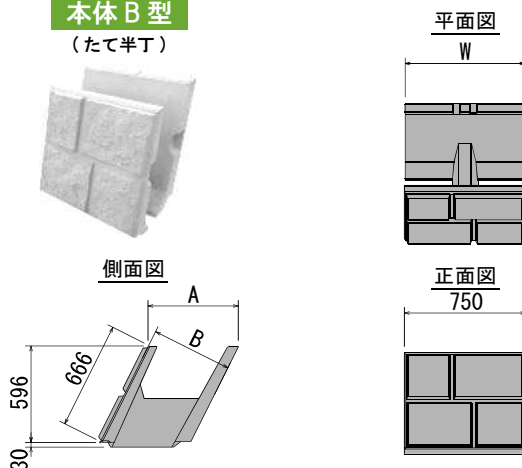
本体 B 型
