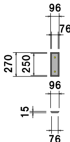
連結部詳細図
