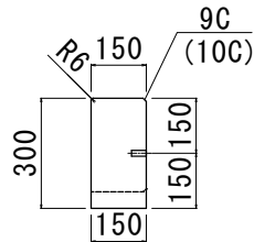
側面図
