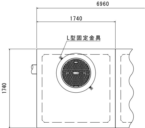
上部(蓋)
