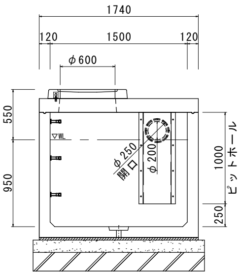
排水ピット (栓付) 詳細図
