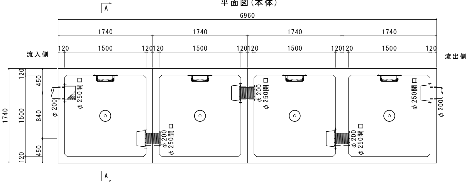
平面図(本体)
