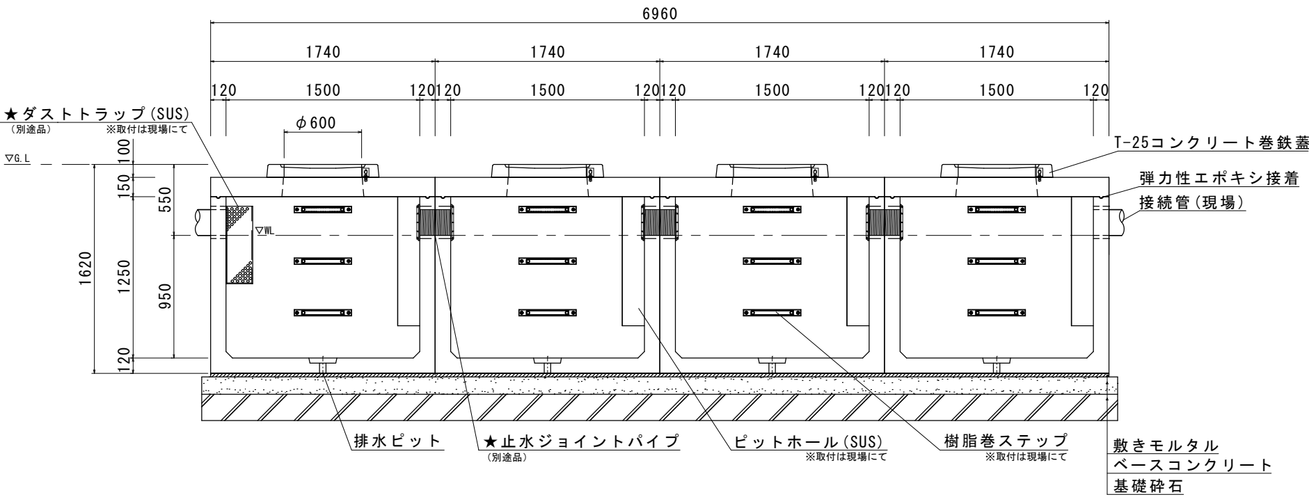
正面断面図
