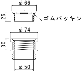
排水ピット (栓付) 詳細図
