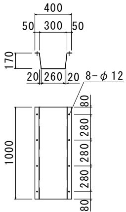
ピットホール(標準)
