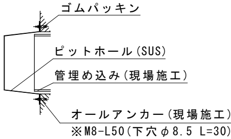
材 料 表 (準備部材) 1200
