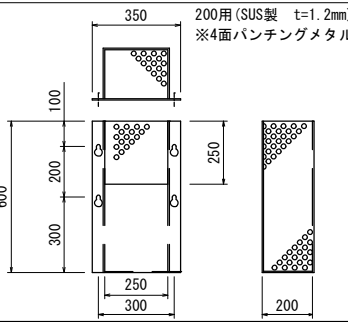
★オプション: 着脱式ダストトラップ
