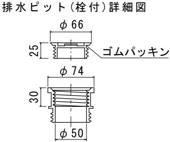
排水ピット (栓付) 詳細図
