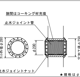
★オプション: 止水ジョイントパイプ
