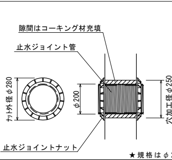
★オプション：止水ジョイントパイプ
