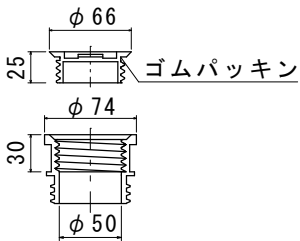
排水ピット (栓付) 詳細図
