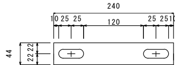
連結プレート t=3.2mm
