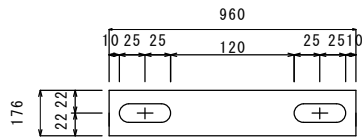
連結プレート t=3.2mm
