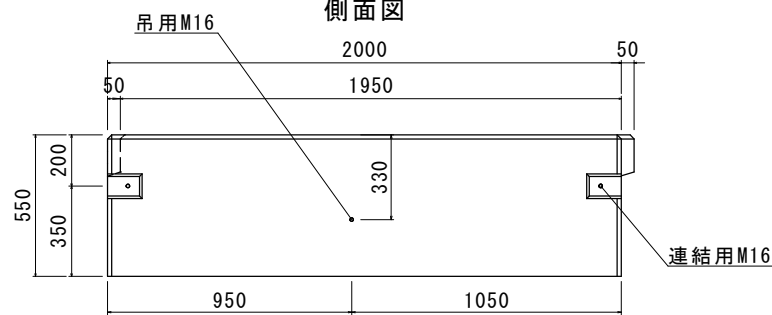
側面図
