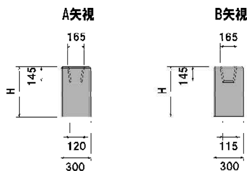
正面図
