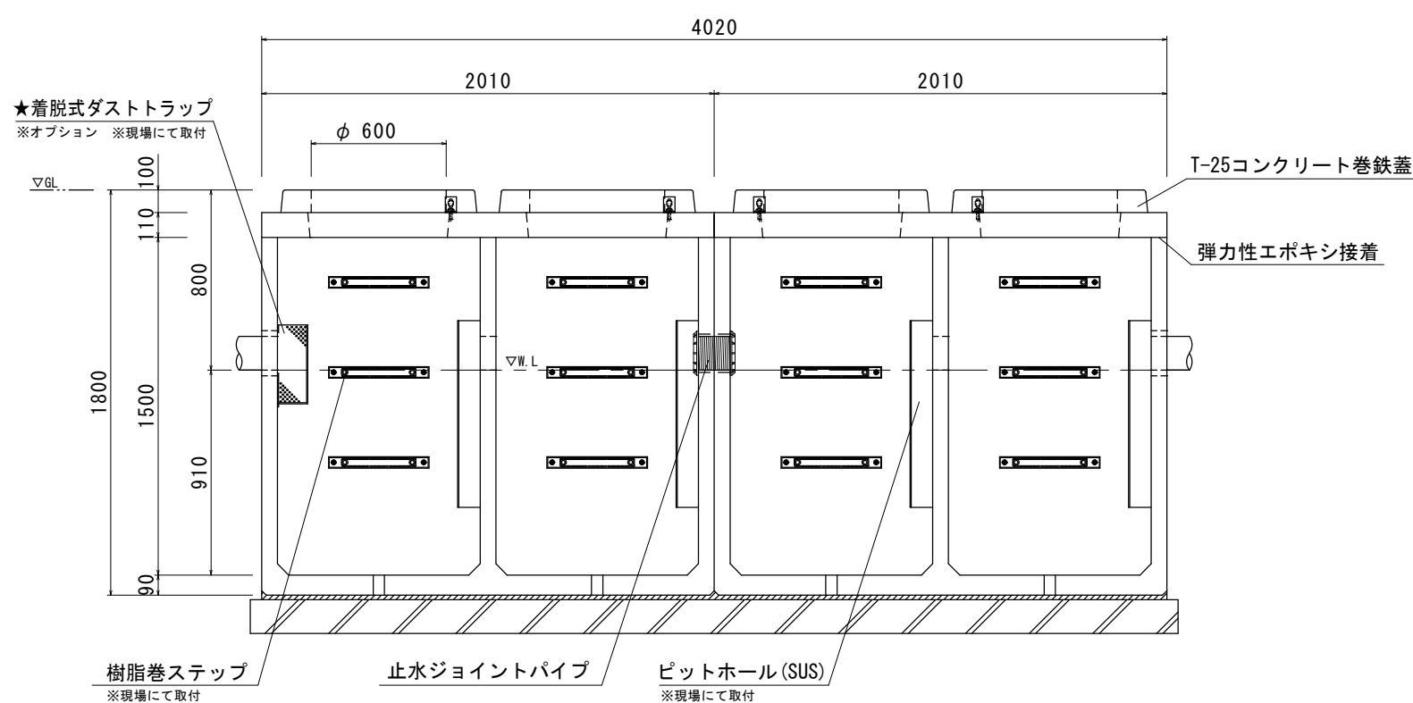
B-B断面図
