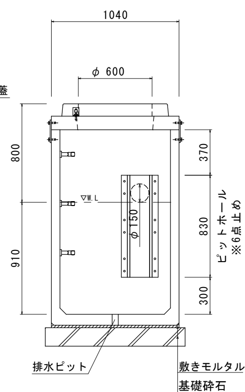
A-A断面図
