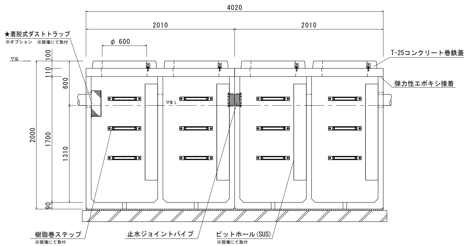
B-B断面図
