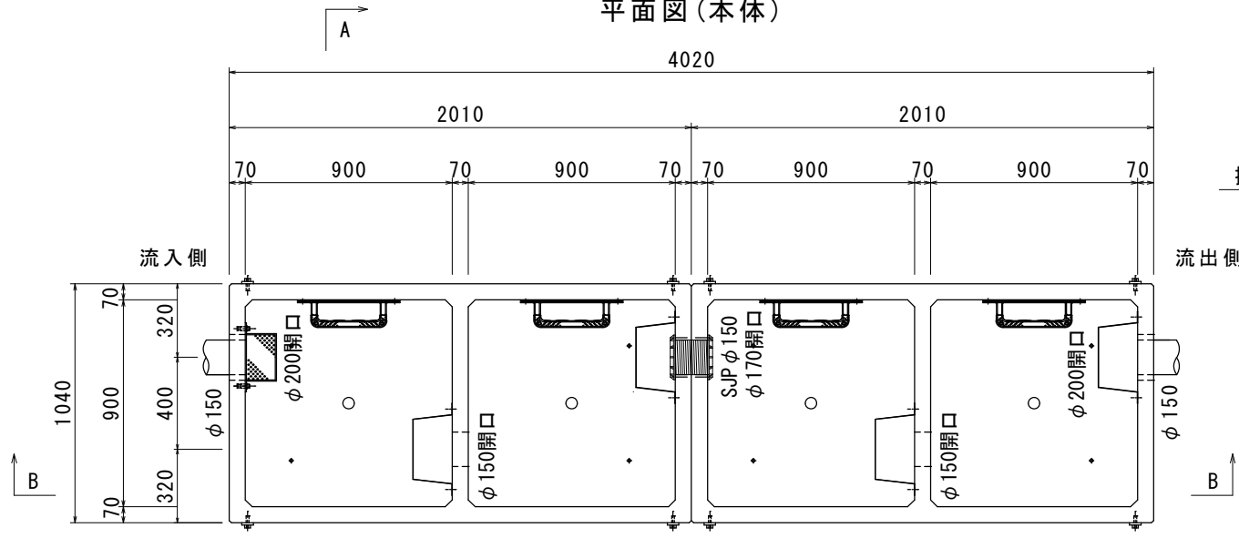
平面図(本体)
