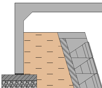
門型カルバート等
