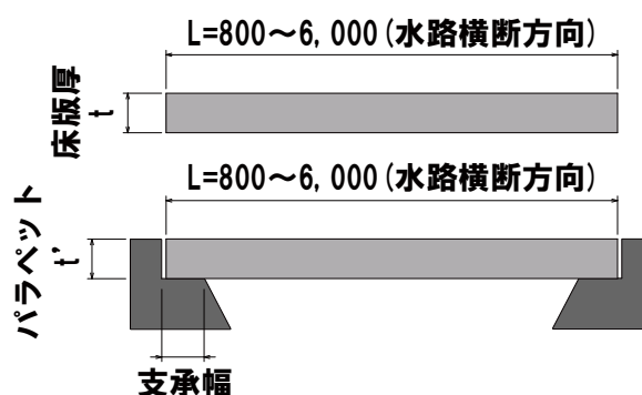
側面図
