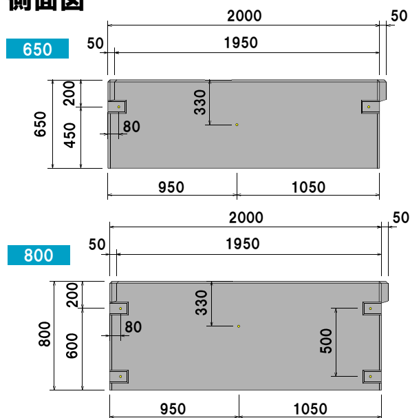
側面図
