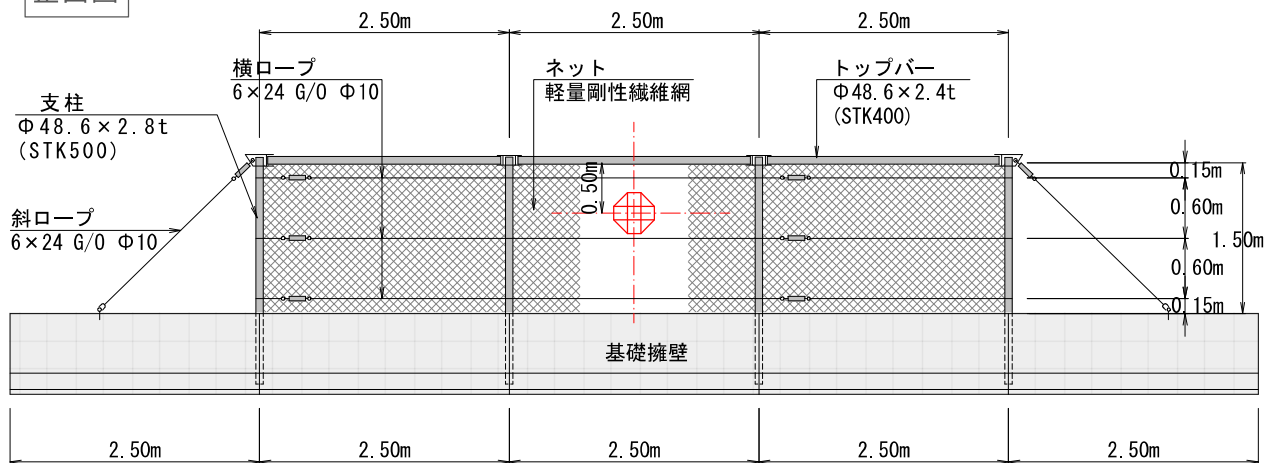
実験供試体の概要図
