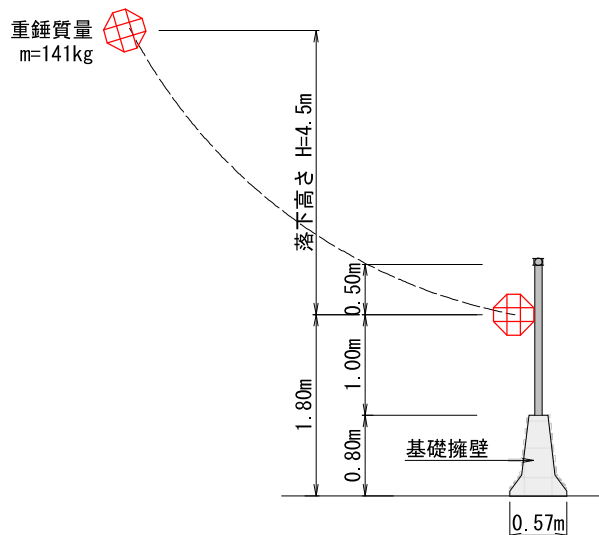
振り子式実験装置の概要図
