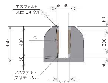
曲線部施工
