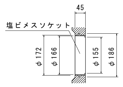
A部詳細図(埋込み部) ※S=1/10
