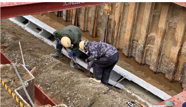
4. 裏込材を入れながら積む (1)
