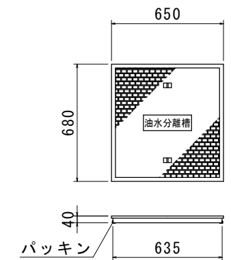
T-25 鑄鐵蓋
