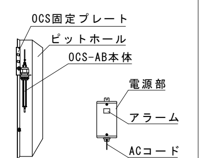
★OCS-AB オイルチェックセンサー
