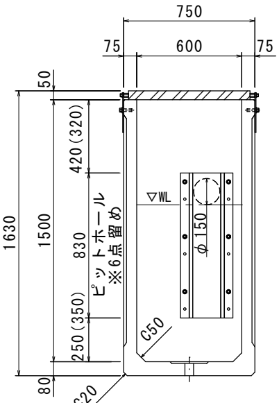
槽内断面図
