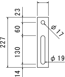
B部詳細図 (埋込み部)
