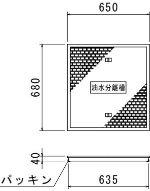
ピットホール取付詳細図
