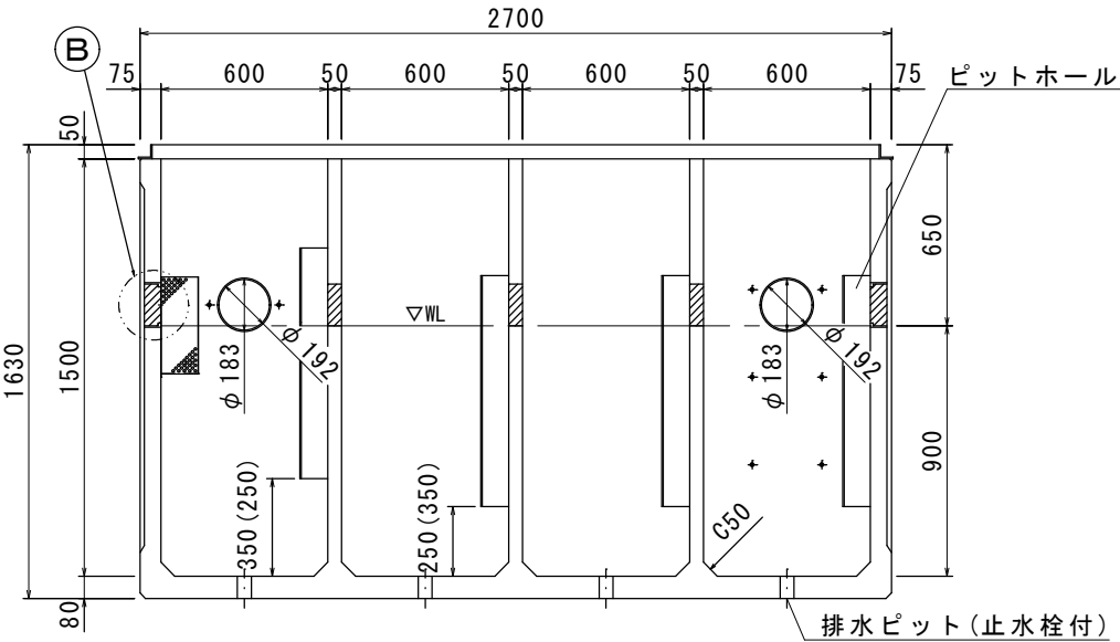
正面図
