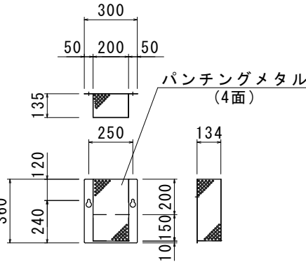
★ダストトラップ SUS
