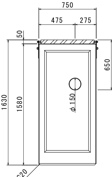
流入側面図
