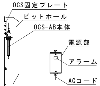
★OCS-AB オイルチェックセンサー
