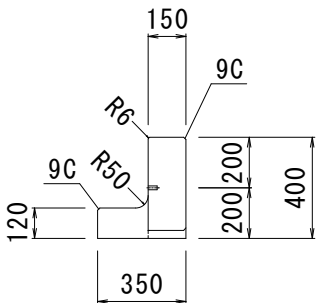
側面図
