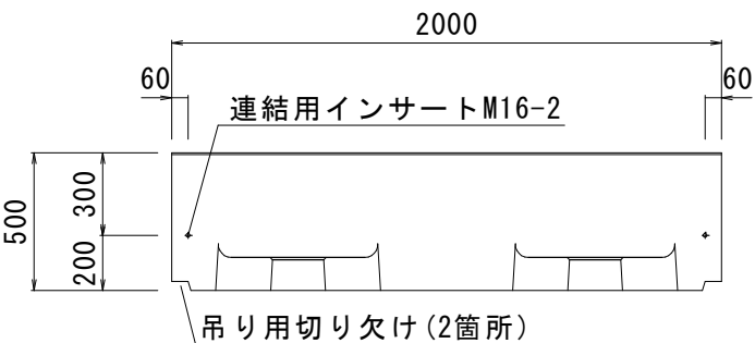
B矢視正面図
