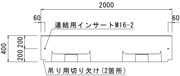
B矢視正面図
