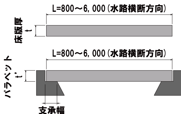
側面図
